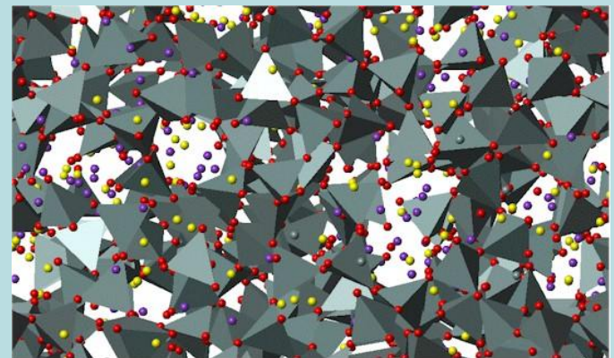
DL_POLY – динамическое полуэмпирическое моделирование
